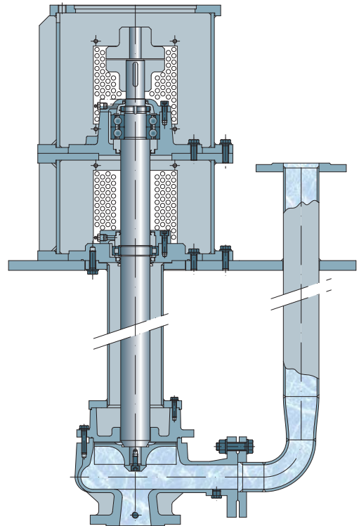
CANTILEVER LONGITUDINAL SECTION CANTILEVER SEZIONE LONGITUDINALE
