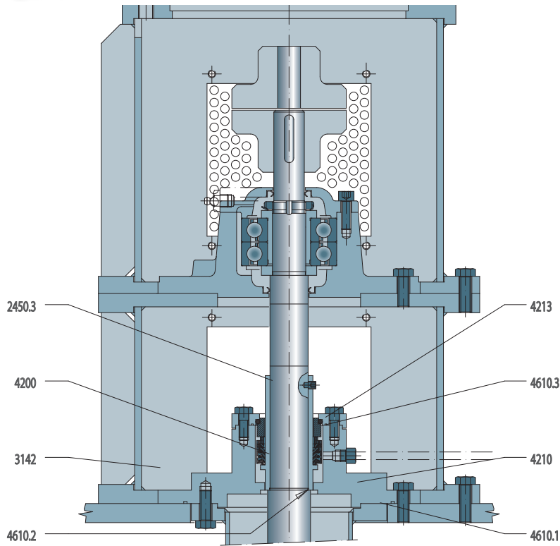
MECHANICAL SEAL VERSION VERSIONE TENUTA MECCANICA
